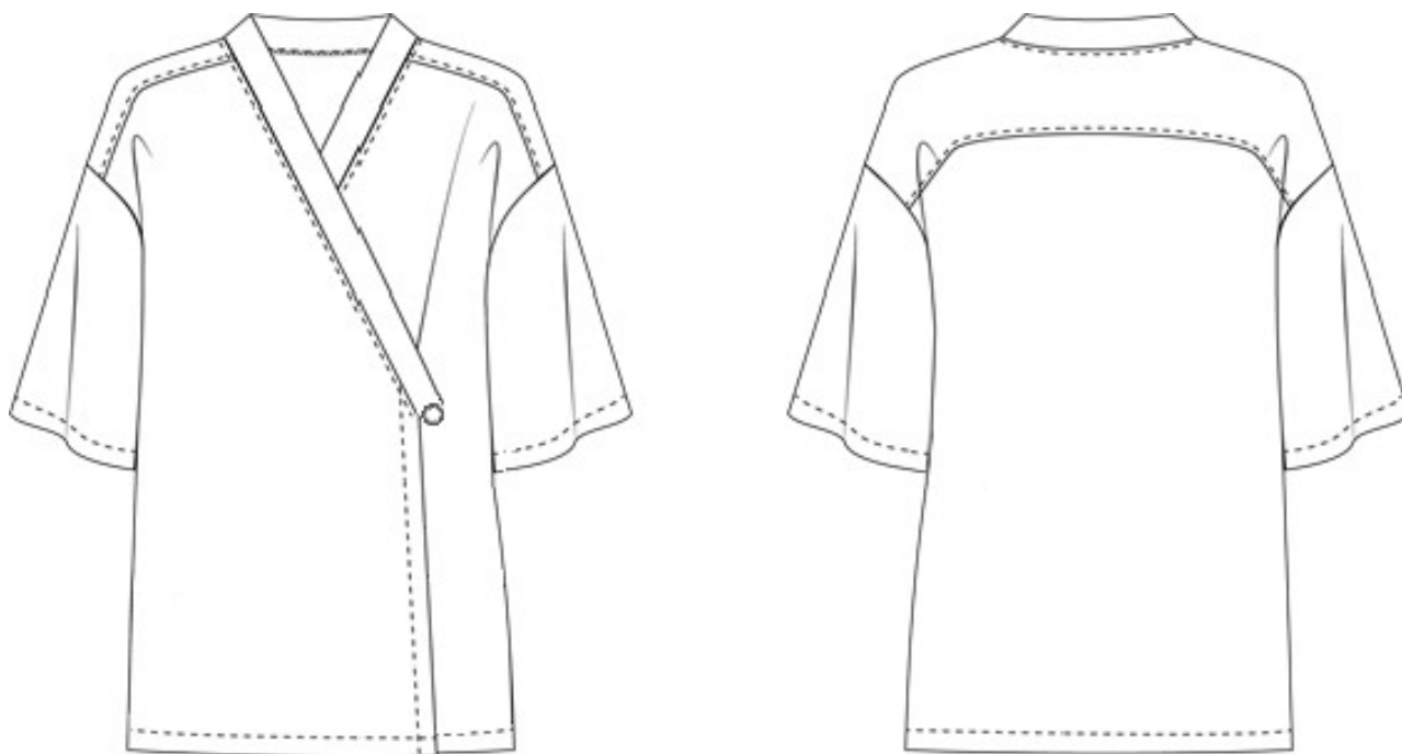
Рисунок 2 – Технический рисунок женской блузы.
